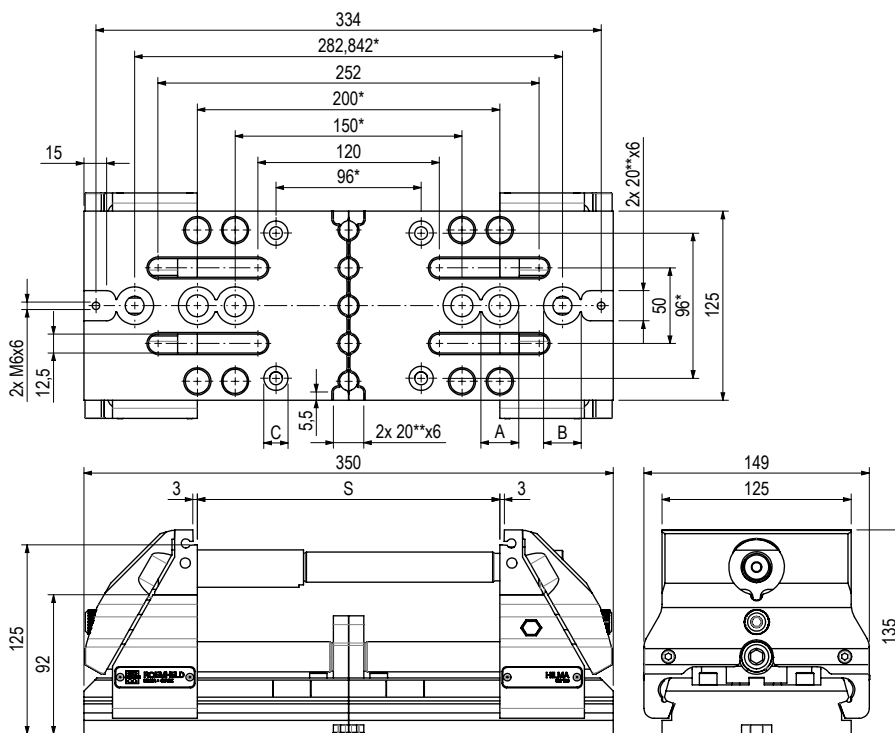
Abbildung: 970230101 Standard Lieferumfang: Maschinen-Schraubstock inkl. Niederzug-Spannbacken, Spannmutter kurz und lang, Zugspindel kurz und lang
