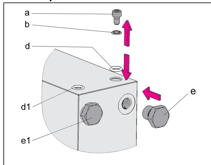
Fig. 9: Ejemplo, preparación para el montaje con conexión hidráulica sin tuberías
