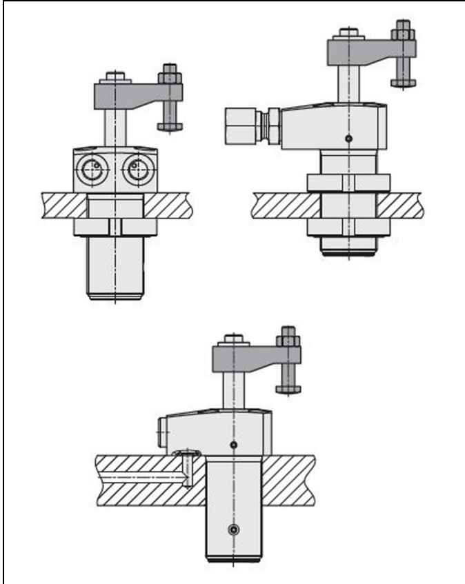
Fig. 3: Brida arriba
