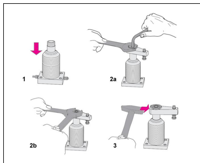
Fig. 10: Montaje / desmontaje - ejemplo
