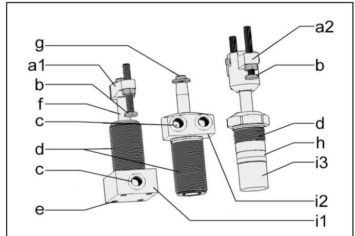
Fig. 1: Componentes
