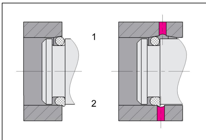
Fig. 8: Instalación a través de chaflán de entrada y orificio transversal
