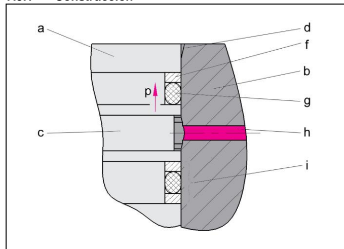
Fig. 7: Componentes
