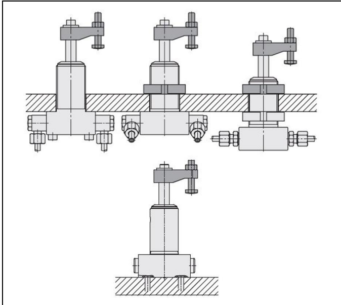
Fig. 4: Brida abajo
