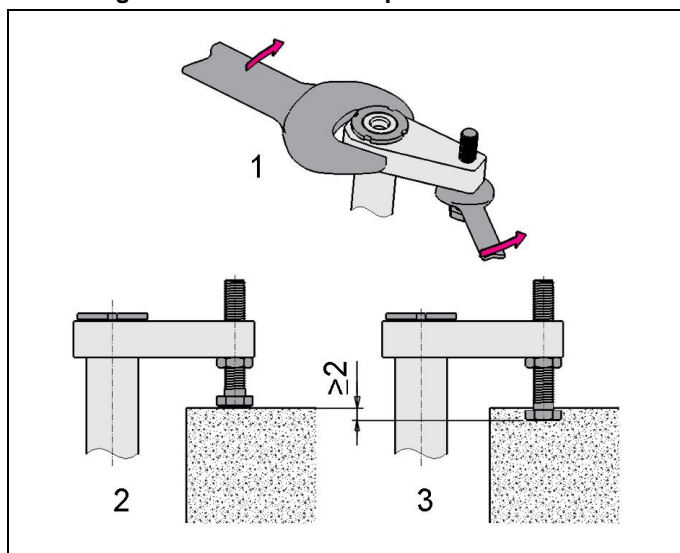
Fig. 11: Regulación de la brida de sujeción - ejemplo
