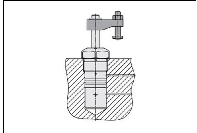
Fig. 5: Ejecución enroscable
