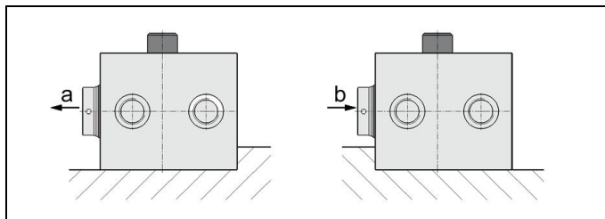
Fig. 4: Vérin-bloc appuyé
