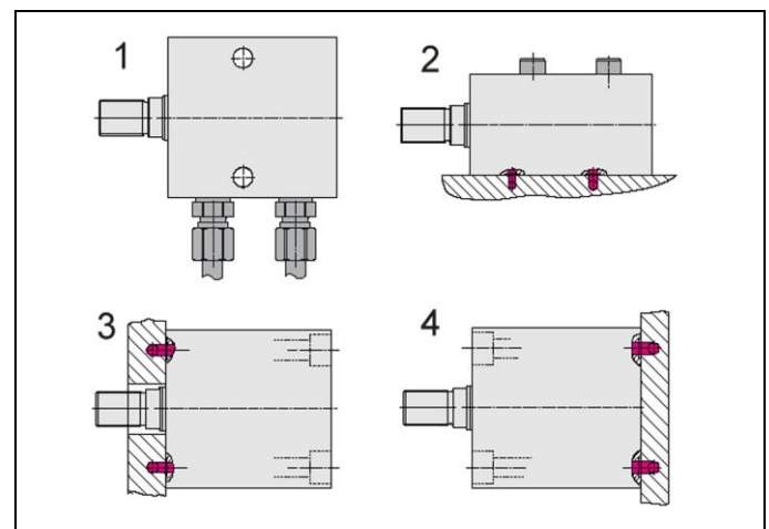
Fig. 3: Types de connexion de l'alimentation en huile hydraulique
