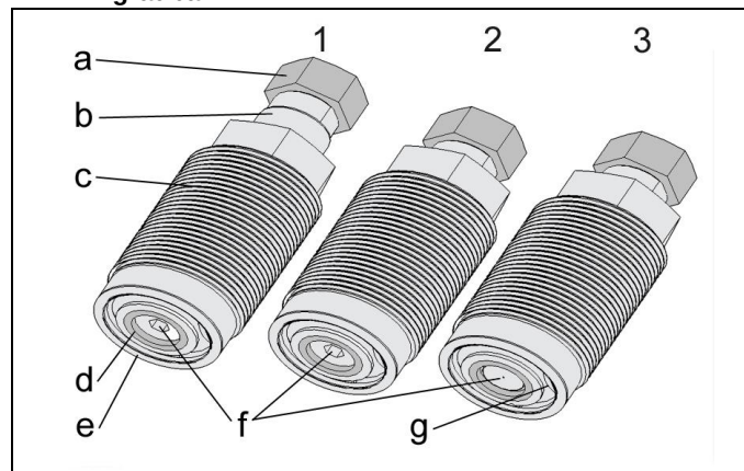
Slika 1: sestavni deli
