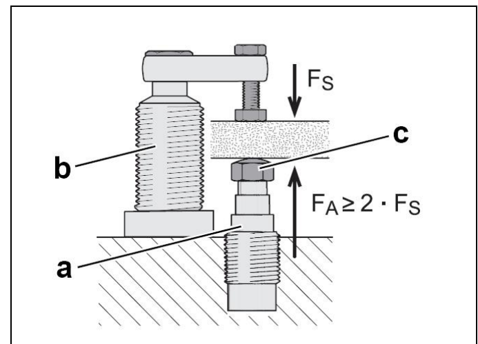
Fig. 2: Principio, flujo de fuerzas durante el apoyo
