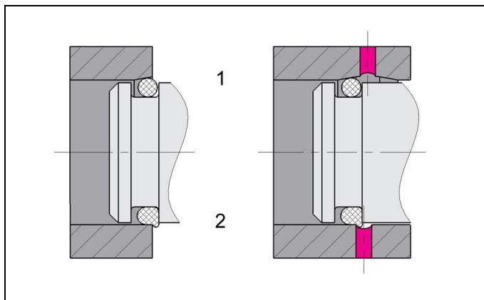
Fig. 5: Installation par chanfrein d'entrée et alésage transversal
