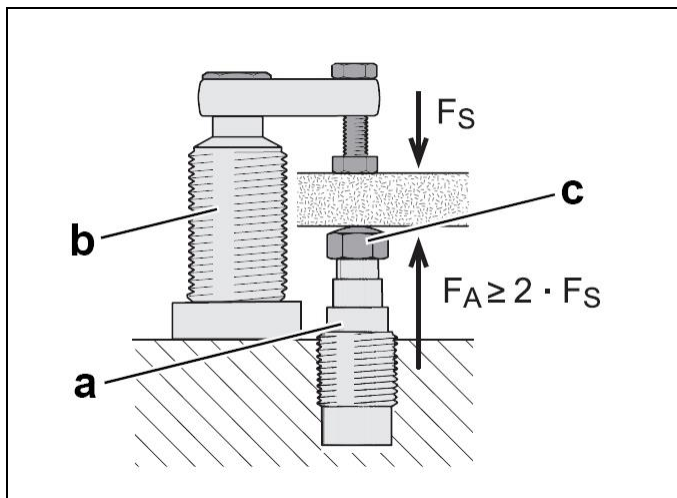
2. ábra: Alapelv, teljesítményáramlás a támasz során
