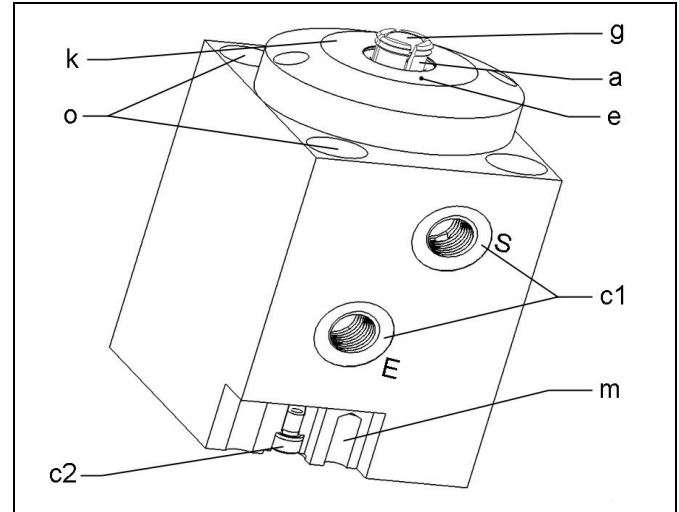
Fig. 1: Componentes
