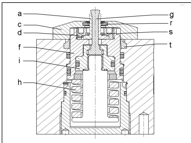
Fig. 5: Componentes
