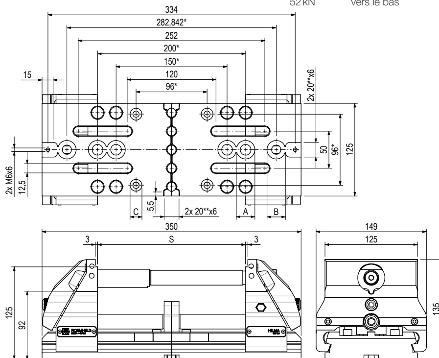
Mécanisme de traction vers le bas
