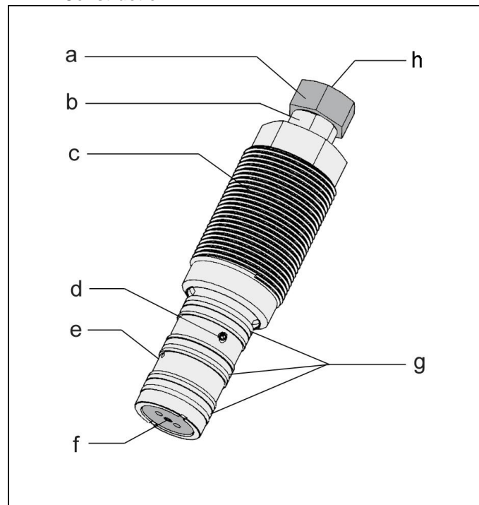
Fig. 1 : Composants
