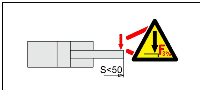
Fig. 5: Introduire les forces transversales
