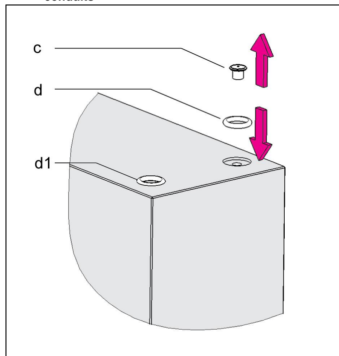
Fig. 7 : Exemple, préparation pour des connexions hydrauliques sans tuyauterie
