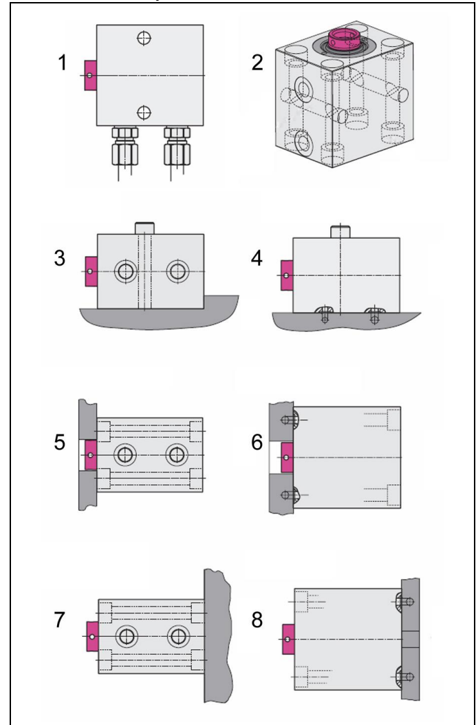
Fig. 2: Possibilités de fixation
