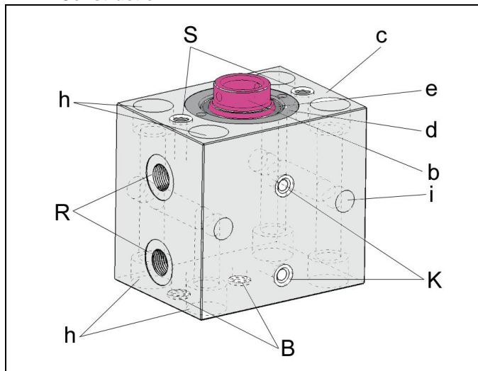
Fig. 1: Schéma de principe des composantes et des connexions
