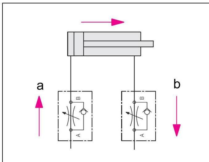
Fig. 6: Schéma hydraulique avec étrangleurs
